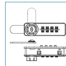
Mechanikus számszár
